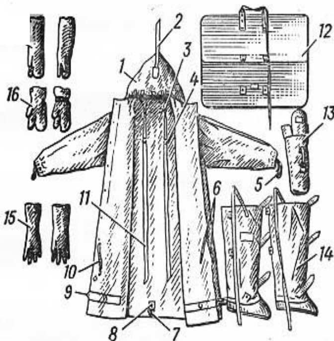
Рис. 6.1. Общевойсковой защитный комплект:
